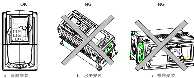
图 4.1 变频器安装方向
