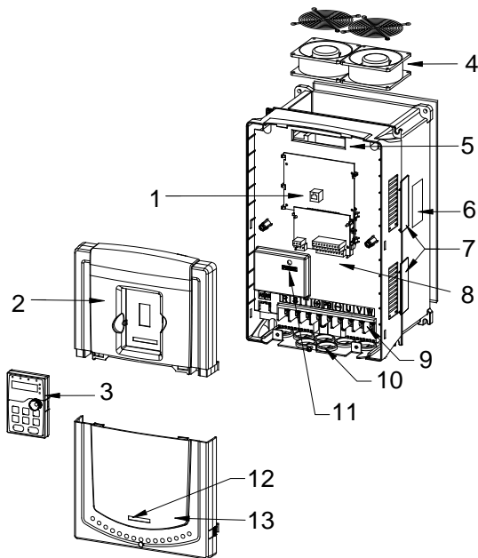
图 3.5 产品结构示意图
