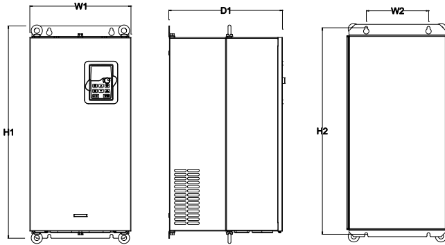
图 B.5 037G/045P~110G/132P 壁挂安装示意图
