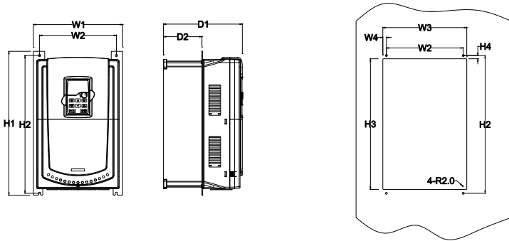
图 B.9 018G/022P~030G/037P 法兰安装示意图
