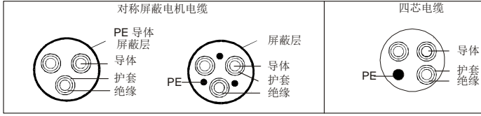
图 C.1 对称屏蔽电机电缆
