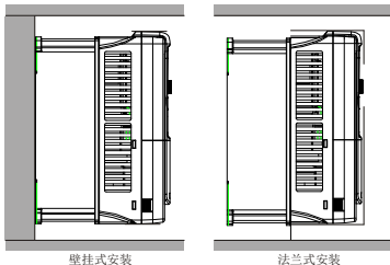
图 4.2 安装方式
