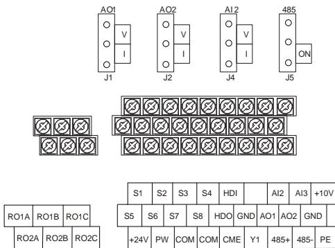
图 4.20 015G/018P 及以下控制端子示意图
