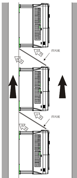
图 4.4 垂直安装
