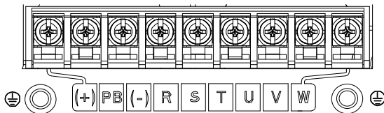
图 4.9 0R7G-5R5G/7R5G 主回路端子示意图
