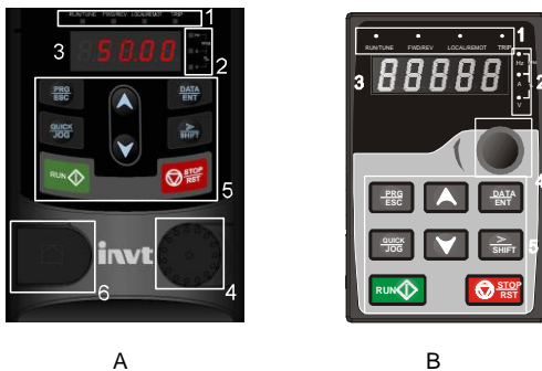
图 5.1 键盘示意图
