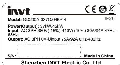
图 3.3 产品铭牌
