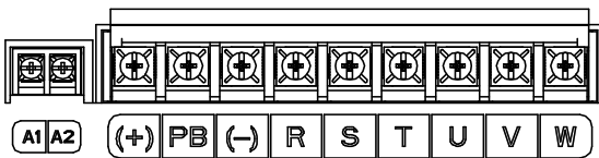
图 4.11 018G/022P 主回路端子示意图
