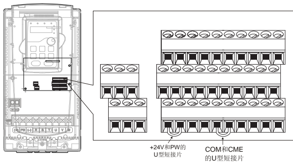
图 4.22 U 型短接位置示意图
