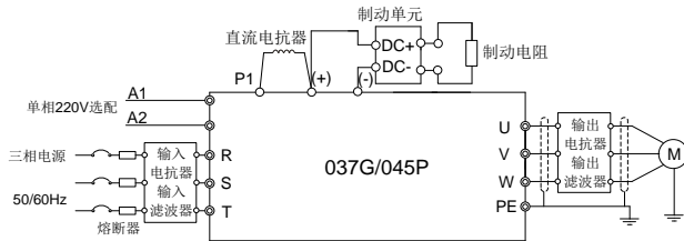
图 4.8 037G/045P 及以上主回路接线图
