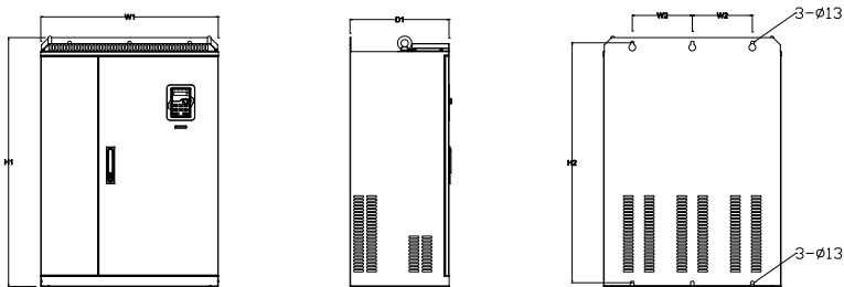
图 B.7 220G/250P~315G/355P 壁挂安装示意图
