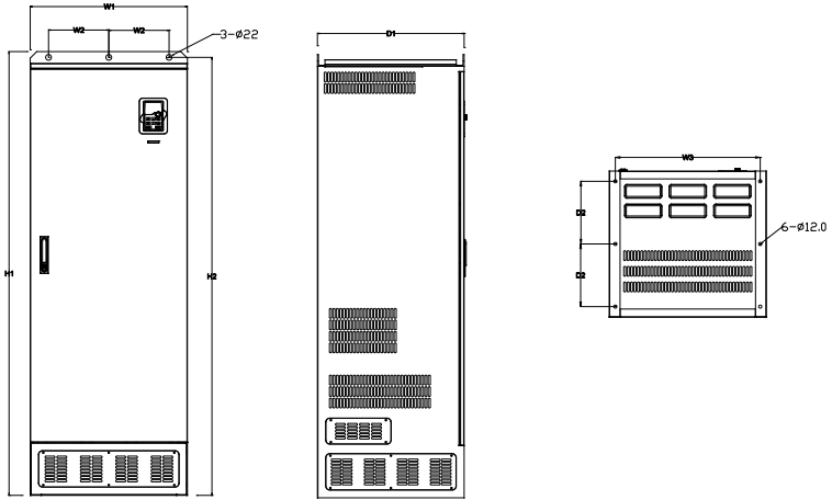
图 B.13 355G/400P~500G 落地安装示意图
