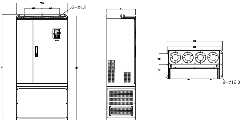
图 B.12 220G/250P~315G/355P 落地安装示意图
