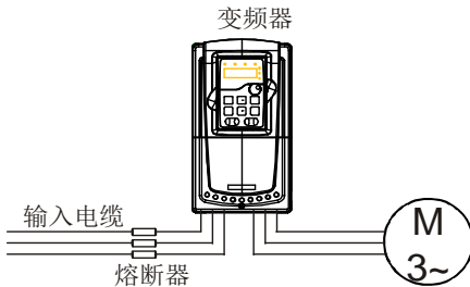
图 4.25 熔断器配置图
