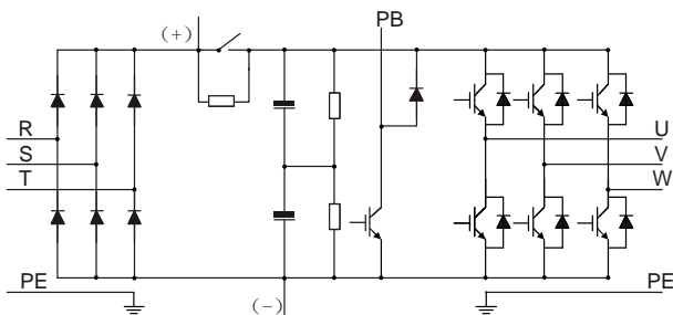
图 3.1 030G/037P 及以下主回路简图
