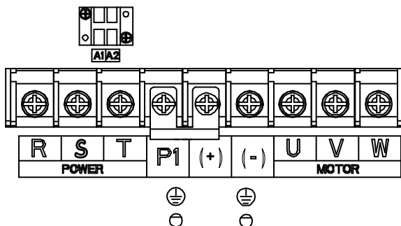
图 4.13 037G/045P~055G/075P 主回路端子示意图
