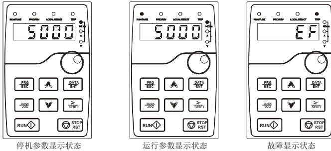
图 5.2 状态显示示意图
