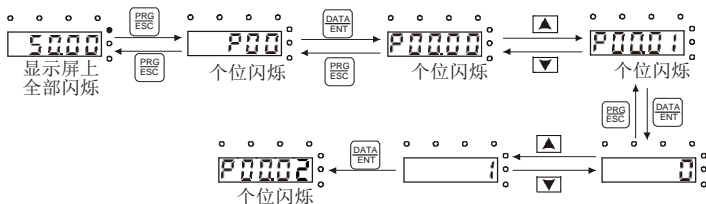
图 5.3 修改参数示意图
