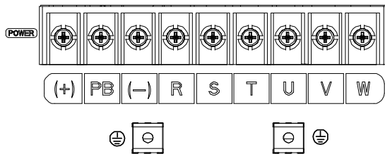
图 4.10 7R5G/011P-015G/018P 主回路端子示意图
