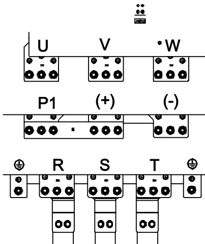
图 4.17 355G/400P~500G 主回路端子示意图
