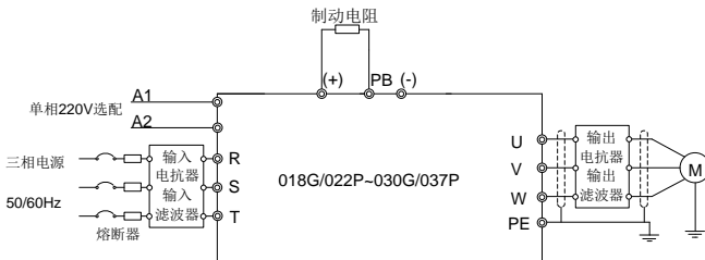
图 4.7 018G/022P-030G/037P 主回路接线图
