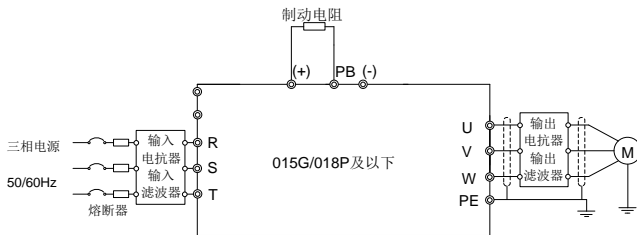
图 4.6 015G/018P 及以下主回路接线图
