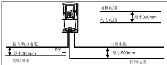
图 C.4 布线距离
