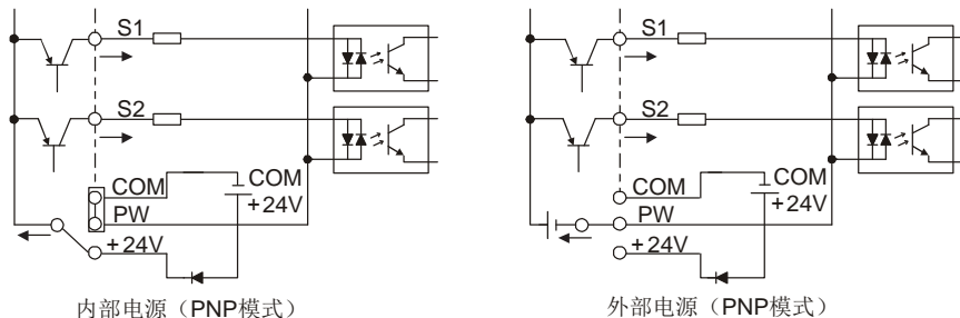
图 4.24 PNP 模式示意图
