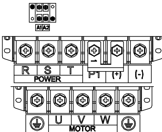
图 4.14 075G/090P~110G/132P 主回路端子示意图
