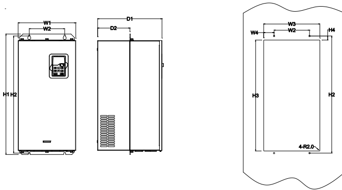
图 B.10 037G/045P~110G/132P 法兰安装示意图
