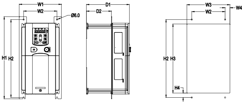
图 B.8 0R7G~015G/018P 法兰安装示意图
