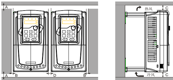
图 4.3 并行安装
