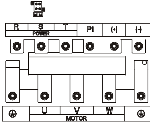
图 4.15 132G/160P~200G/220P 主回路端子示意图
