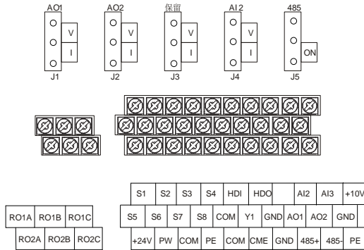
图 4.21 018G/022P 及以上控制端子示意图
