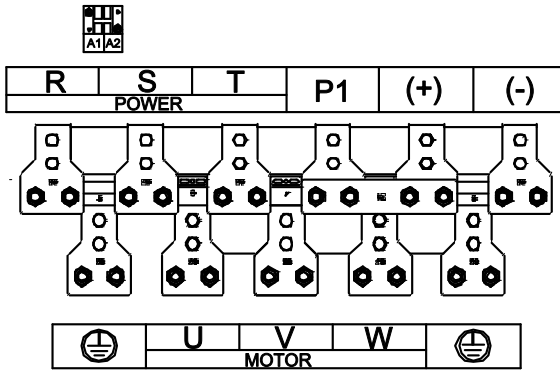
图 4.16 220G/250P~315G/355P 主回路端子示意图
