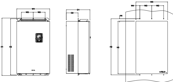
图 B.11 132G/160P~200G/220P 法兰安装示意图
