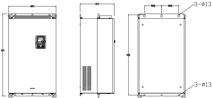
图 B.6 132G/160P~200G/220P 壁挂安装示意图
