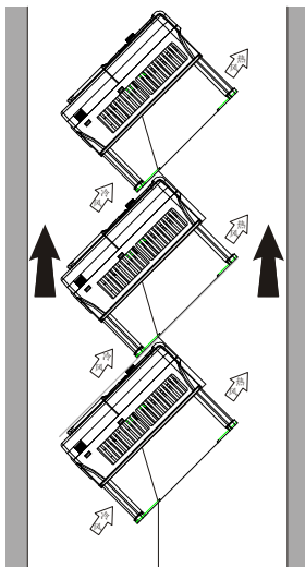
图 4.5 倾斜安装
