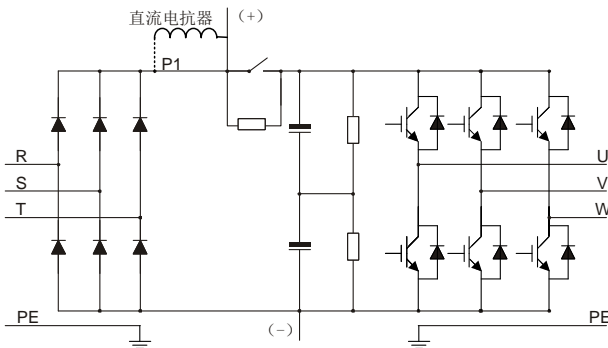
图 3.2 037G/045P 及以上主回路简图
