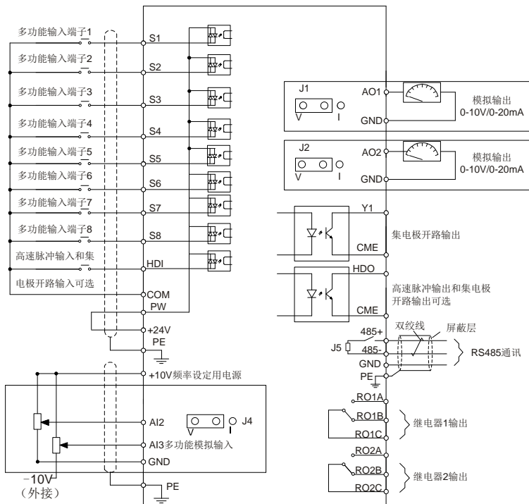
图 4.19 控制回路接线图
