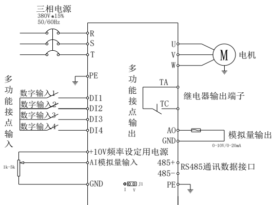
图 3-5 控制回路接线图
