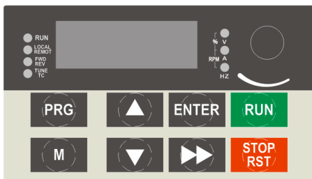
图 4-1 操作面板示意图
