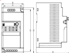
图 6-1 4KW-11KW 变频器外形尺寸示意图
