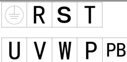
图 3-5 7.5kW-11kW（2030 型）主回路接线端子
